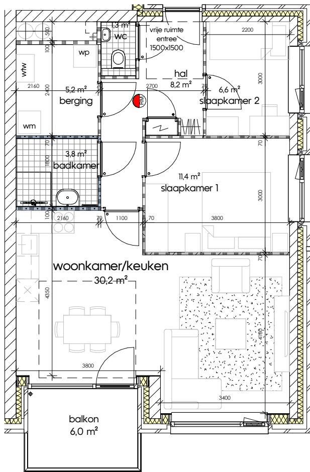
TYPE D | 3-kamer GO 69,4 m 2
